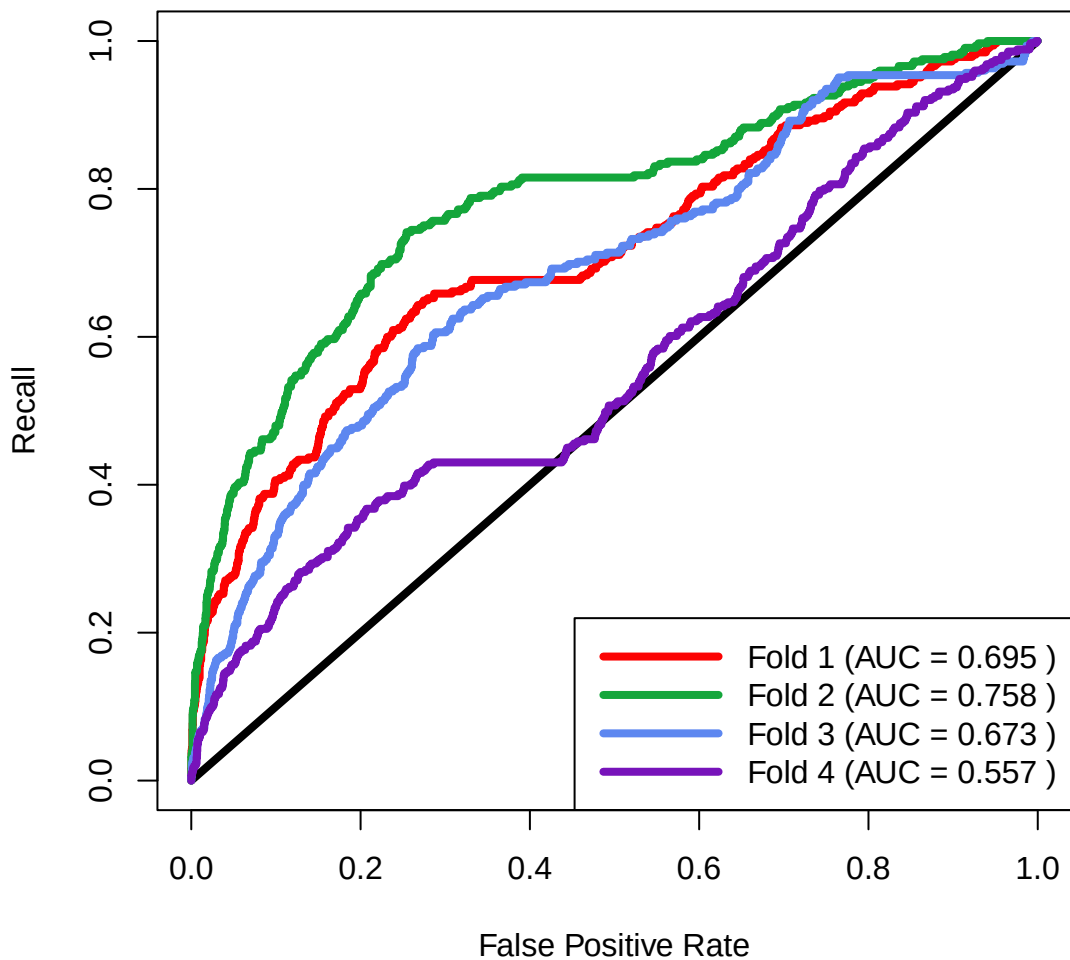
SPELL All Datasets: 430x20x1 Run 1
